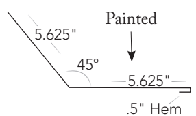
8 Endwall
