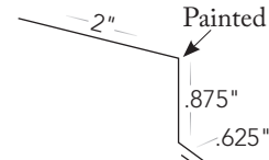
20 Drip Edge Drip Edge
