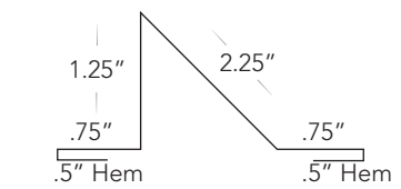
15 Mini Carolina Snow Guard
