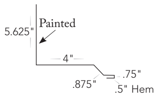
6 Sidewall
