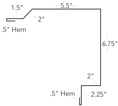
Rake #R-RT
