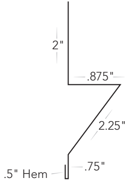
Reglet Flashing #S-RF
