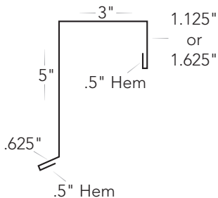
Rake #S-RT
