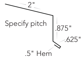
Drip Edge #T-DE
